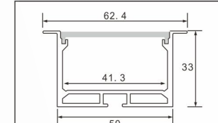
型号: 地踩5032A/52页
