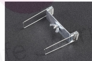
7公分卡簧(嵌装开孔用)
