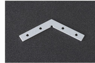
120度连接片 50mm*10mm*2mm 内六角M4螺丝
